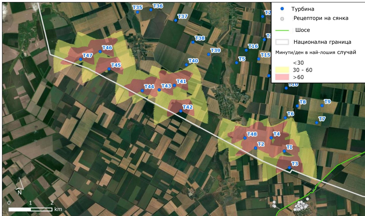
ФИГУРА 5 НАЙ-ЛОШИЯТ СЛУЧАЙ, КАРТА НА ПЕРИОДИЧНОТО ЗАСЕНЧВАНЕ (МИНУТИ/ДЕН)
