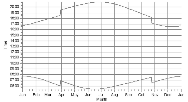
12: VESTAS V170-6.4 6400 170.0 !O! hub: 155.0 m (TOT: 240.0 m) (24)
