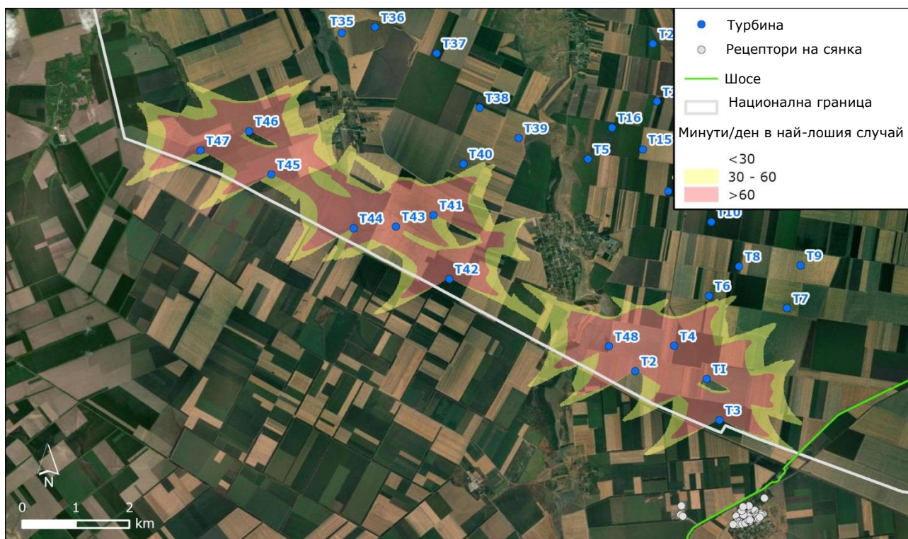
ФИГУРА 5 НАЙ-ЛОШИЯТ СЛУЧАЙ, КАРТА НА ПЕРИОДИЧНОТО ЗАСЕНЧВАНЕ (ЧАСОВЕ/ГОДИНА)
