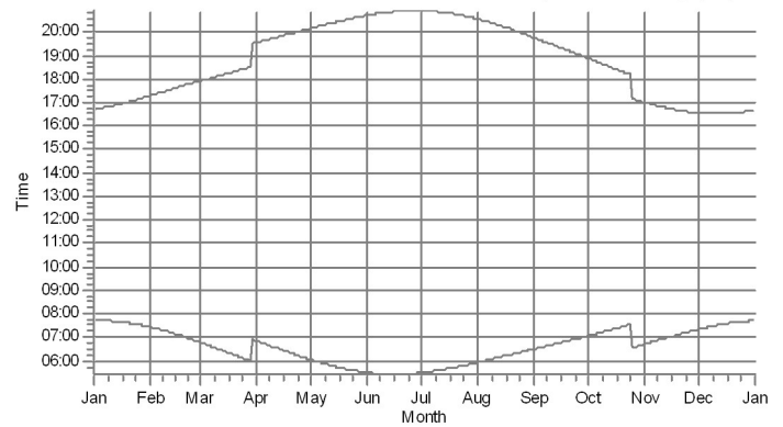
4: VESTAS V170-6.4 6400 170.0 !O! hub: 155.0 m (TOT: 240.0 m) (16)
